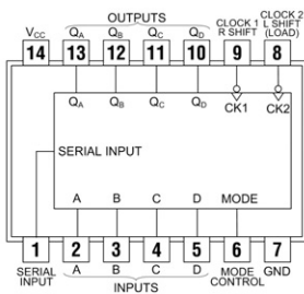
7495 4-Bit Shift Register PIPO
