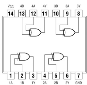
74136 Quad 2-Input XOR O.C.
