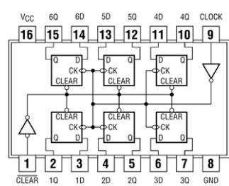
74174 Hex D-Type Flip Flops
